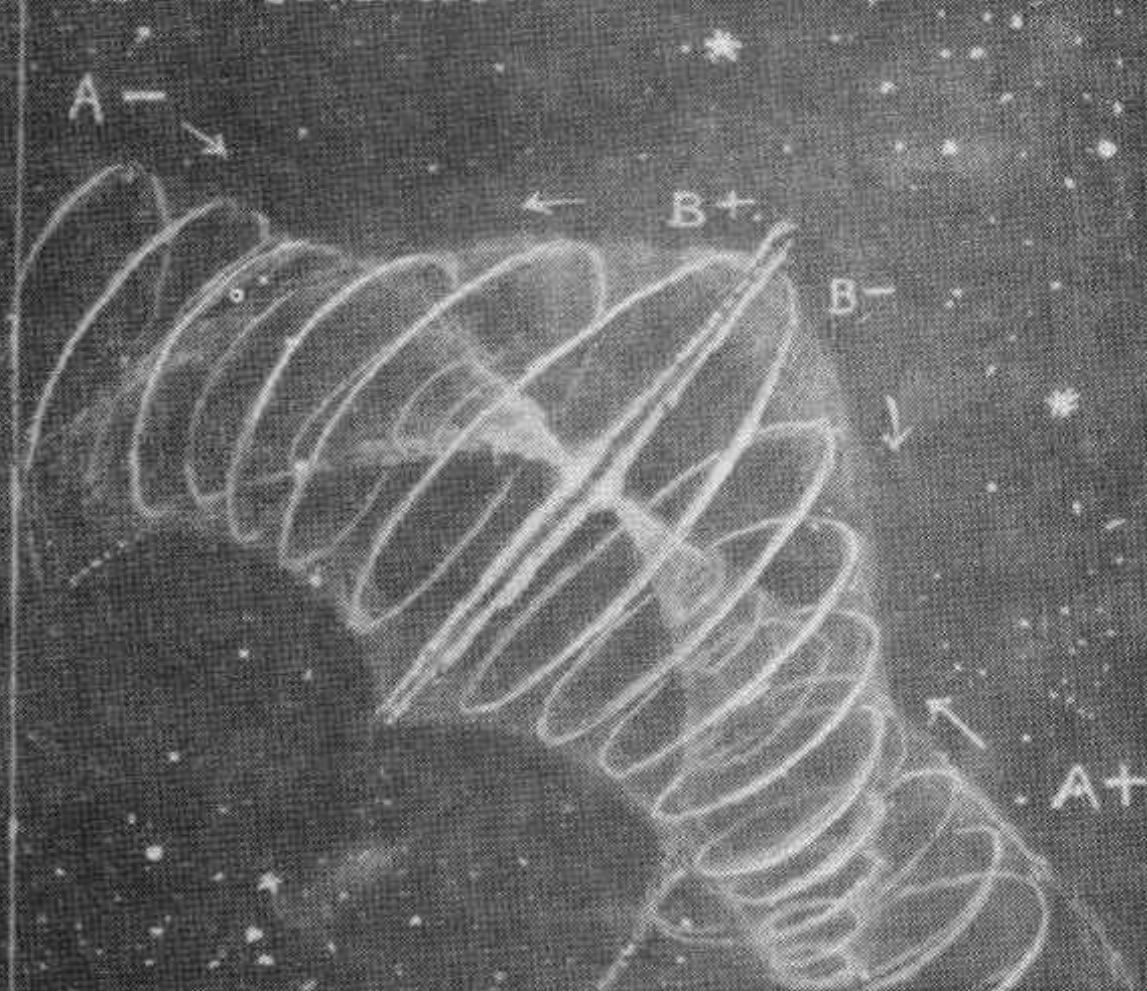
H. V. L. CAMELOPARD FIG. 131. M. 101. URSA MAJOR.
